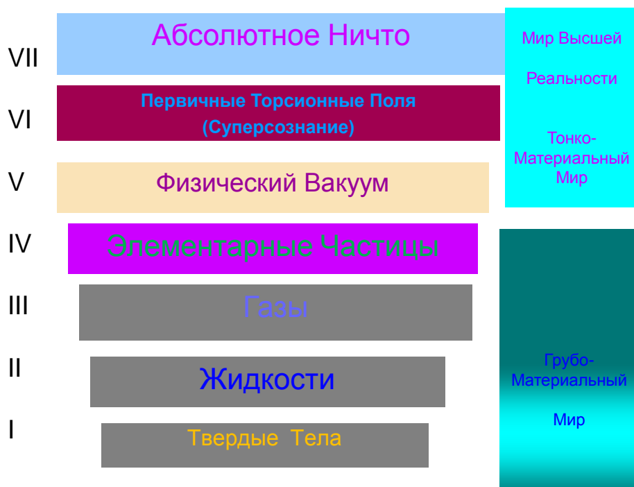
Рис1. Семь Уровней Реальности в Теории Физического Вакуума
