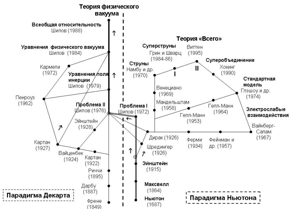
Рис.2. Параллельное развитие двух научных парадигм
